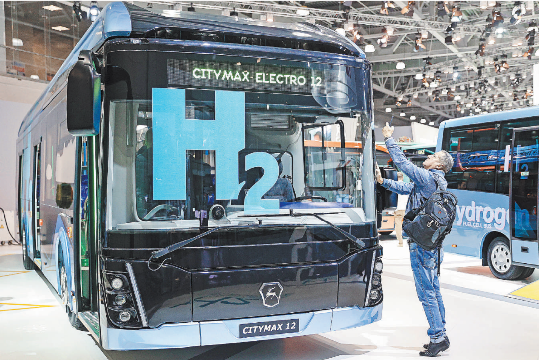
Водоробус Citymax H2 от нижегородского автогиганта ГАЗ способен проехать 350 километров без дозаправки. Фактически его и другой опытный образец от «КАМАЗа», который может проехать без дозаправки до 250 километров, можно использовать и на междугородних маршрутах. Электробусам же приходится после 100 километров автономного хода становиться на зарядку на специализированных станциях.
